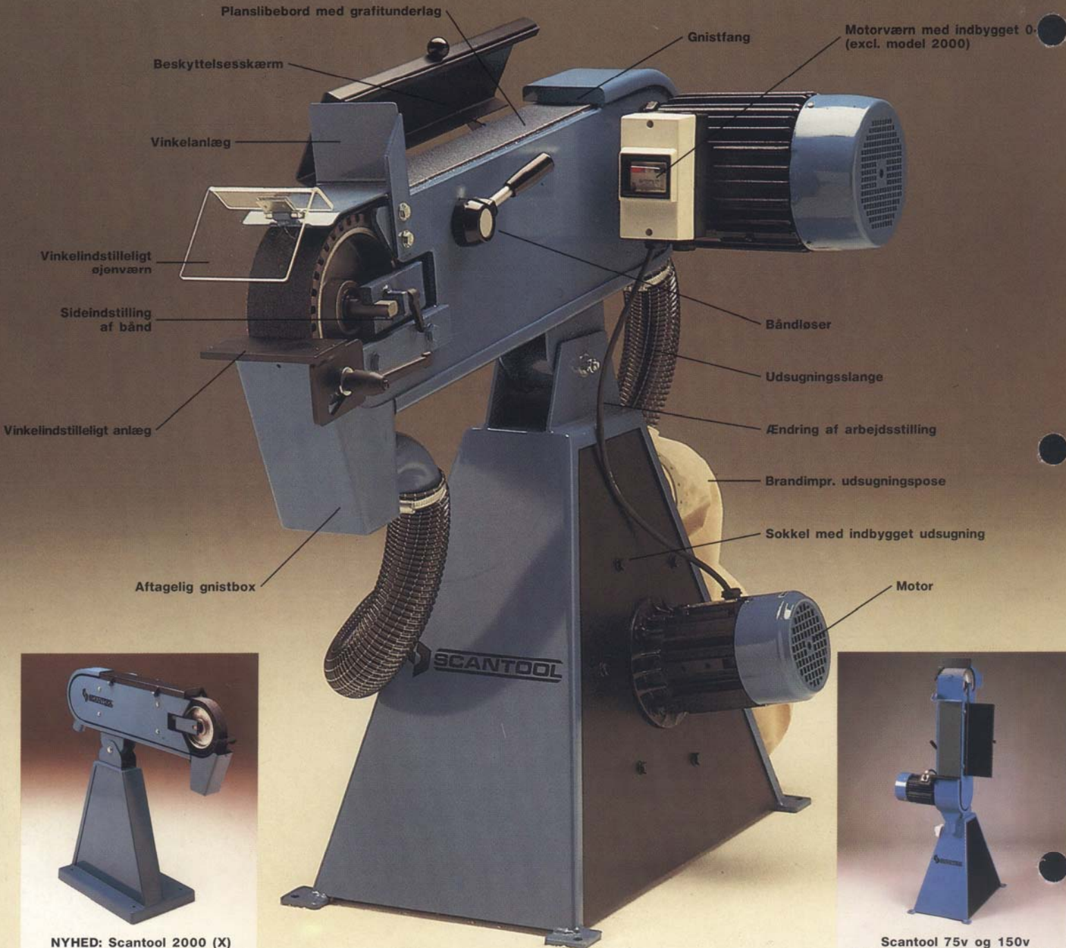
NYHED: Scantool 2000 (X) Værkstedsbåndsliber
